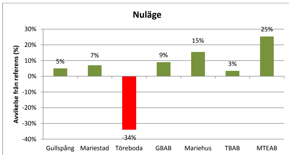
Figur 2: Jämförelse av energiprestandan med Boverkets referensvärde 2009.
